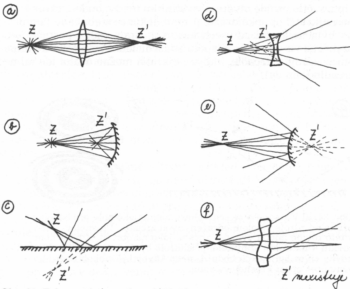
Obr. 35. Zobrazení a) spojkou, b) dutým zrcadlem, c) rovinným zrcadlem, d) rozptylkou, e) vypuklým zrcadlem; f) příklad optické soustavy, která nezobrazuje.
