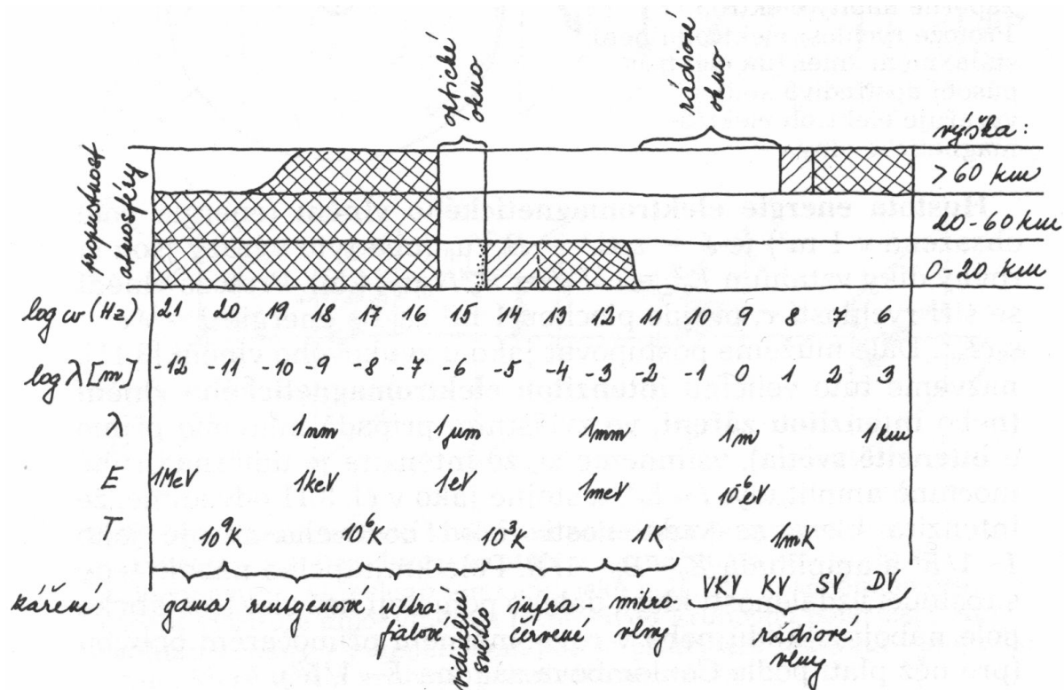
Obr. 28. Rozdělení elektromagnetických vln do spektrálních oborů. Jsou uvedeny frekvence, vlnové délky a pro pozdější odkazy také energie jednoho fotonu a teplota, při níž tělesa vysílají většinu svého záření na této frekvenci. Šrafováním je naznačena propustnost zemské atmosféry v různých výškách nad povrchem.
